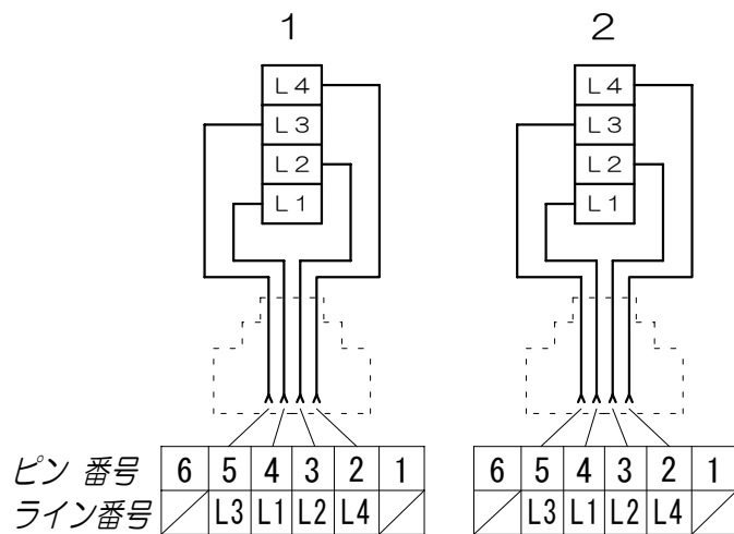
配線図
