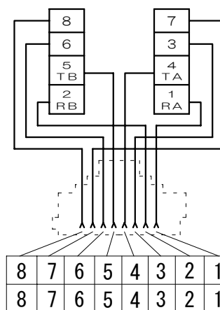
配線図
