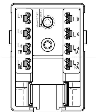
ベース組立図
